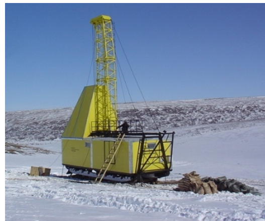
Передвижная буровая установка ПБУ-1200ПП (ПБУ-75СП)
